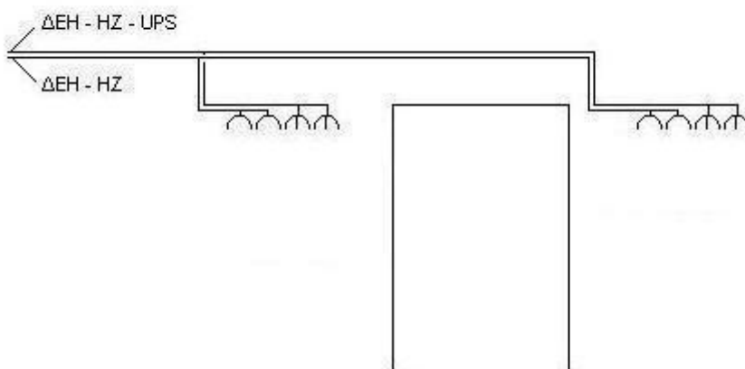
Σχήμα 7.2.6.5 – Διάταξη ρευματοδοτών σε κονσόλα κλίνης ανάνηψης ή χώρου αναζωογόνησης ή πλησίον κεφαλιού κλίνης χώρου γύψου
