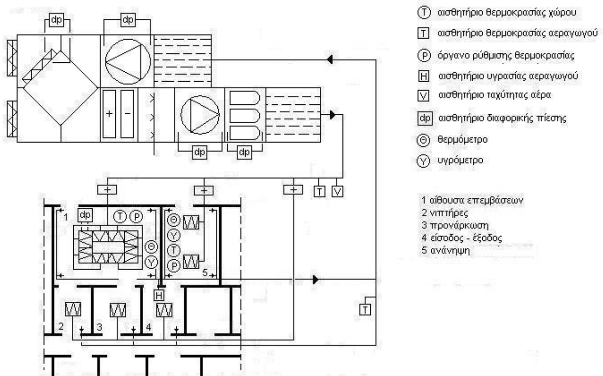
Σχήμα 6.1.9.1.1 – Σύστημα κλιματισμού για 1 αίθουσα επεμβάσεων με τους βοηθητικούς χώρους της και αυτόματος έλεγχος λειτουργίας του συστήματος
