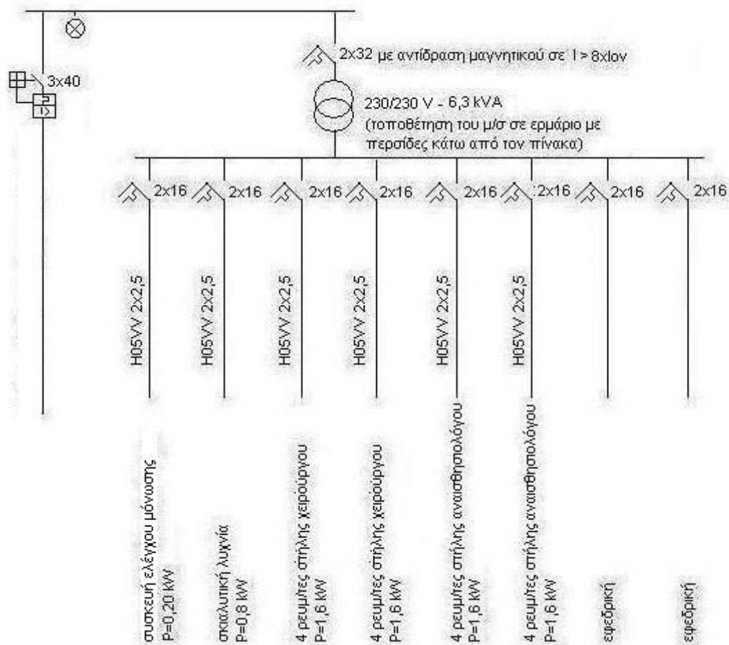
Σχήμα 6.2.6.3 – Ηλεκτρικός πίνακας από ΔΕΗ – ΗΖ – UPS αίθουσας επεμβάσεων
