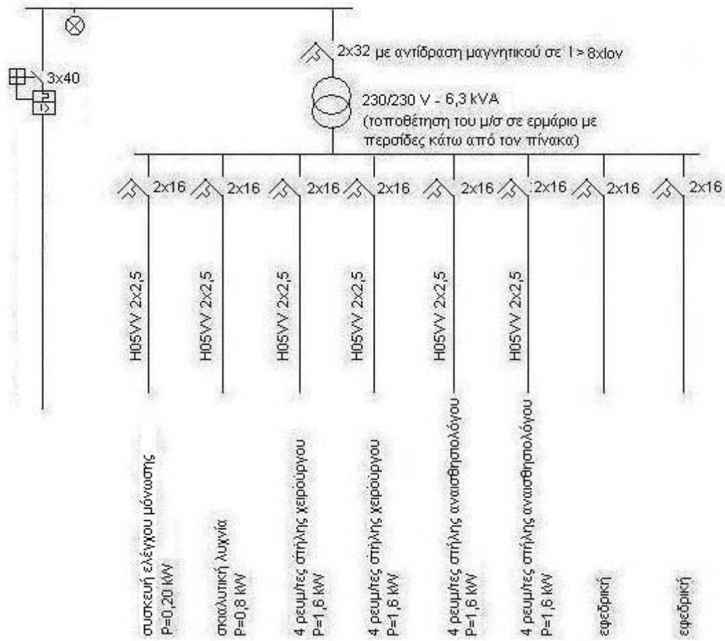
Σχήμα 5.2.6.3 – Ηλεκτρικός πίνακας από ΔΕΗ – ΗΖ – UPS αίθουσας επεμβάσεων
