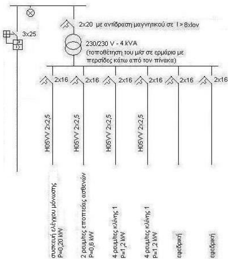
Σχήμα 6.2.6.4 – Ηλεκτρικός πίνακας από ΔΕΗ – ΗΖ – UPS ανάνηψης με 2 κλίνες
