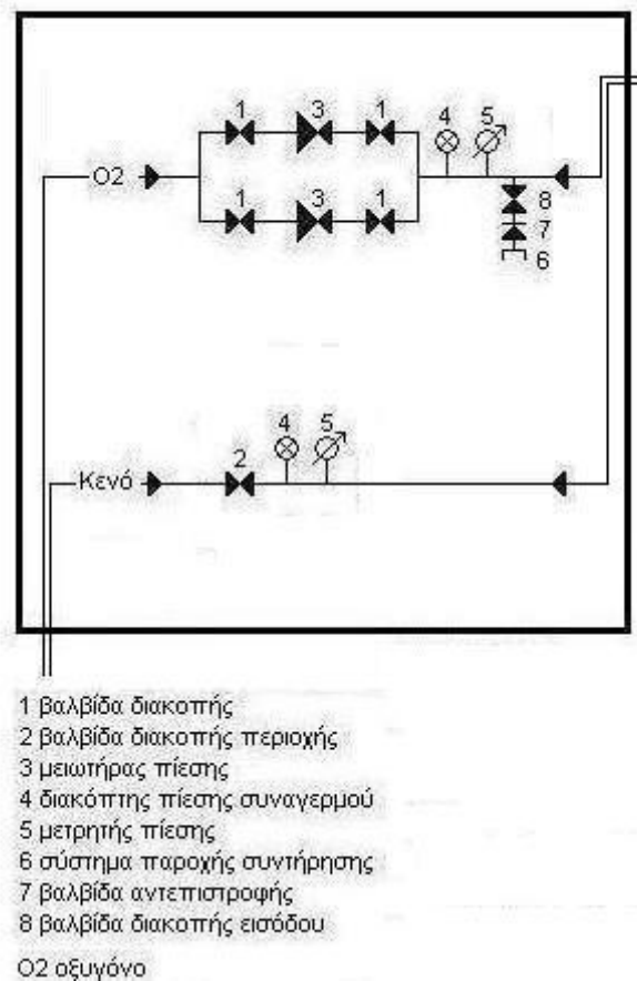
Σχήμα 1.4.3.1 – Σταθμός ελέγχου για μονάδα νοσηλείας
