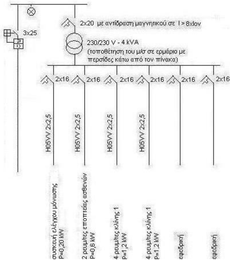
Σχήμα 7.2.6.4 – Ηλεκτρικός πίνακας από ΔΕΗ – ΗΖ – UPS ανάνηψης με 2 κλίνες
