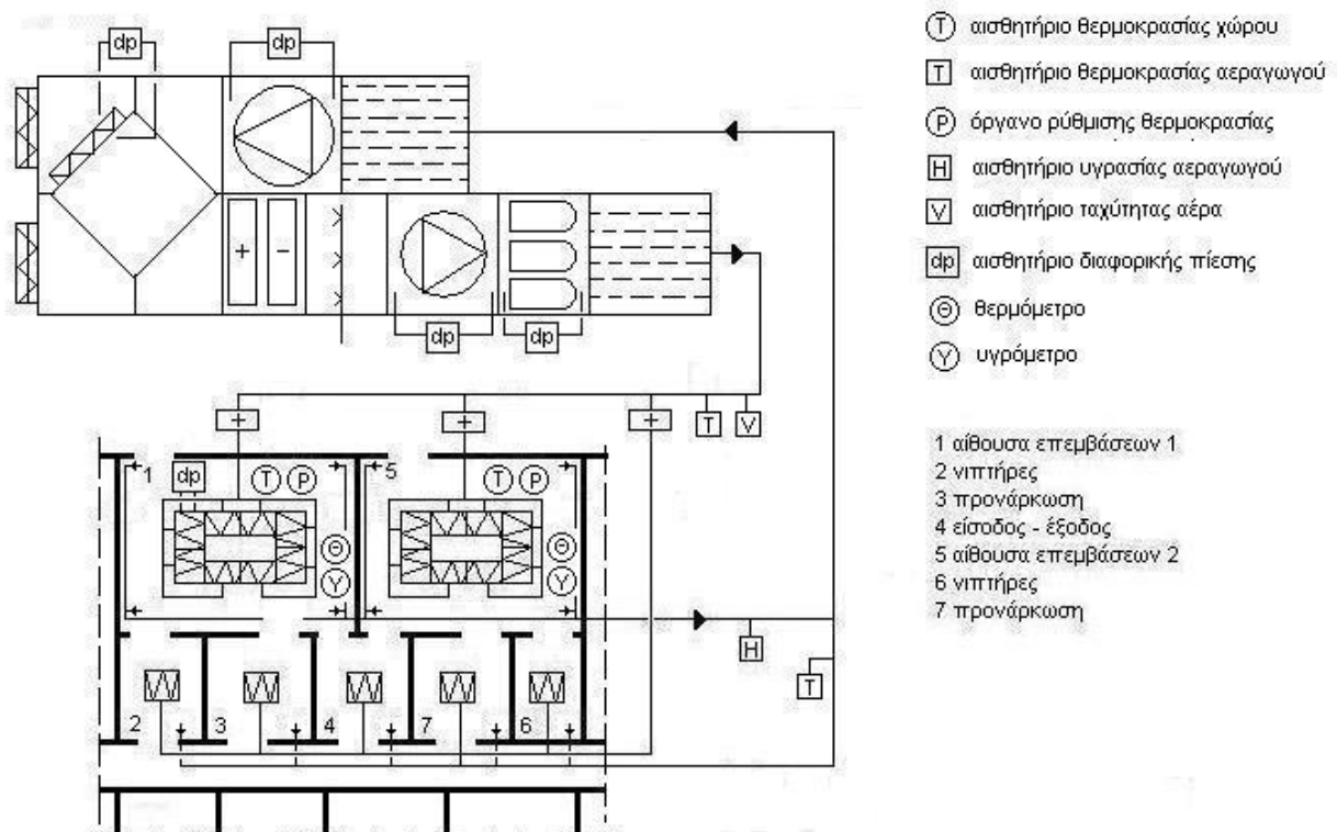
Σχήμα 5.1.9.1.1 – Σύστημα κλιματισμού για 2 αίθουσες επεμβάσεων με τους βοηθητικούς χώρους τους και αυτόματος έλεγχος λειτουργίας του συστήματος
