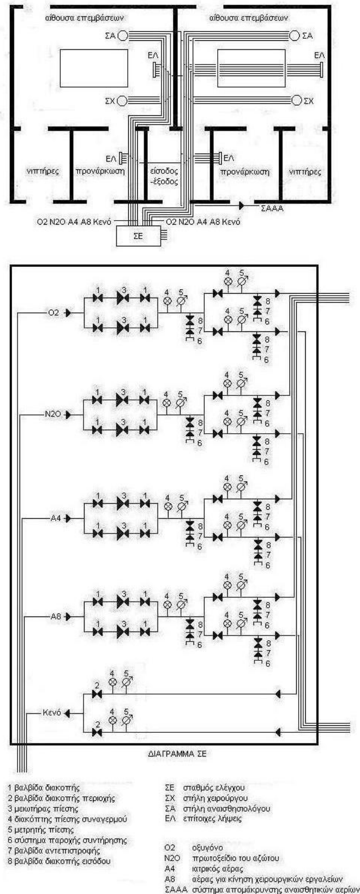
Σχήμα 7.4.3.1 – Σταθμός ελέγχου και δίκτυα για 2 αίθουσες επεμβάσεων με τους βοηθητικούς χώρους τους
