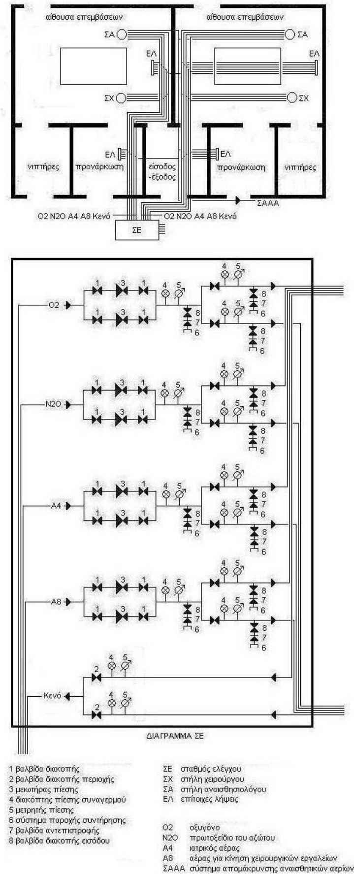
Σχήμα 5.4.3.1 – Σταθμός ελέγχου και δίκτυα για 2 αίθουσες επεμβάσεων με τους βοηθητικούς χώρους τους
