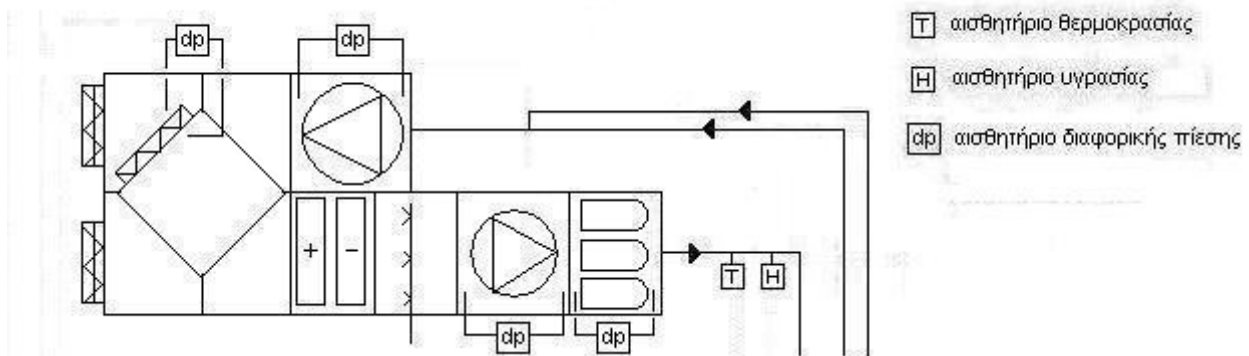
Σχήμα 4.1.9.1 – ΚΚΜ συστήματος κλιματισμού για τμήμα εξωτερικών ιατρείων και αυτόματος έλεγχος λειτουργίας της ΚΚΜ
